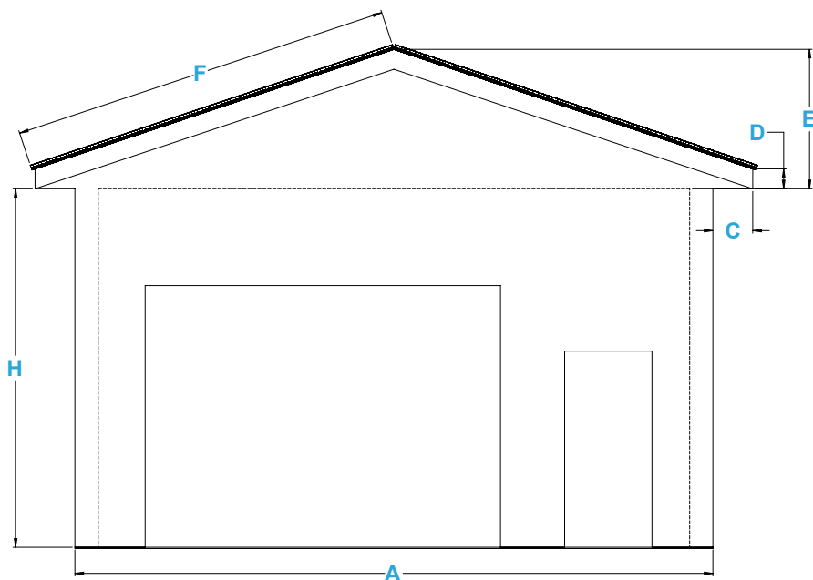
ÉLÉVATION AVANT
